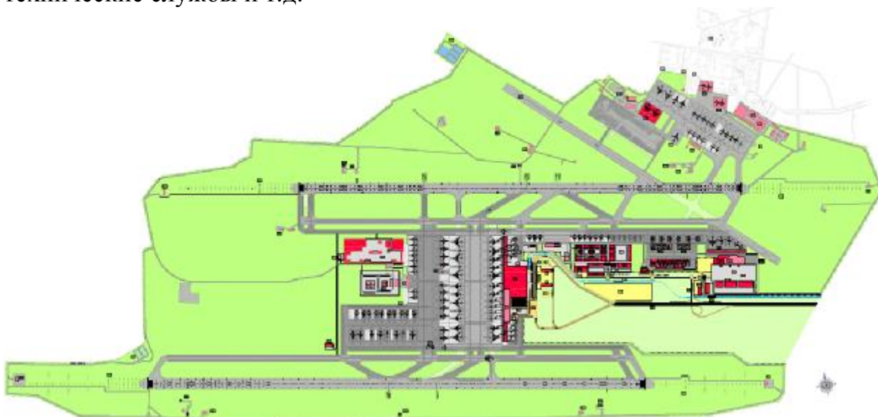
Рис. 1. Генеральный план аэропорта «Пулково»
